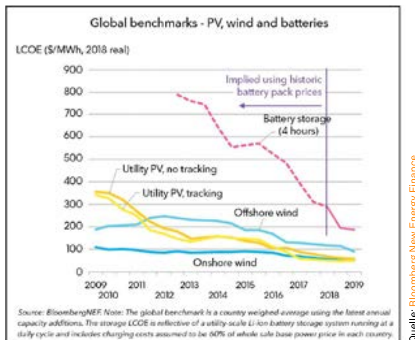
Abb. 3: Kostenentwicklung bei Erneuerbaren Energien und Speichern
